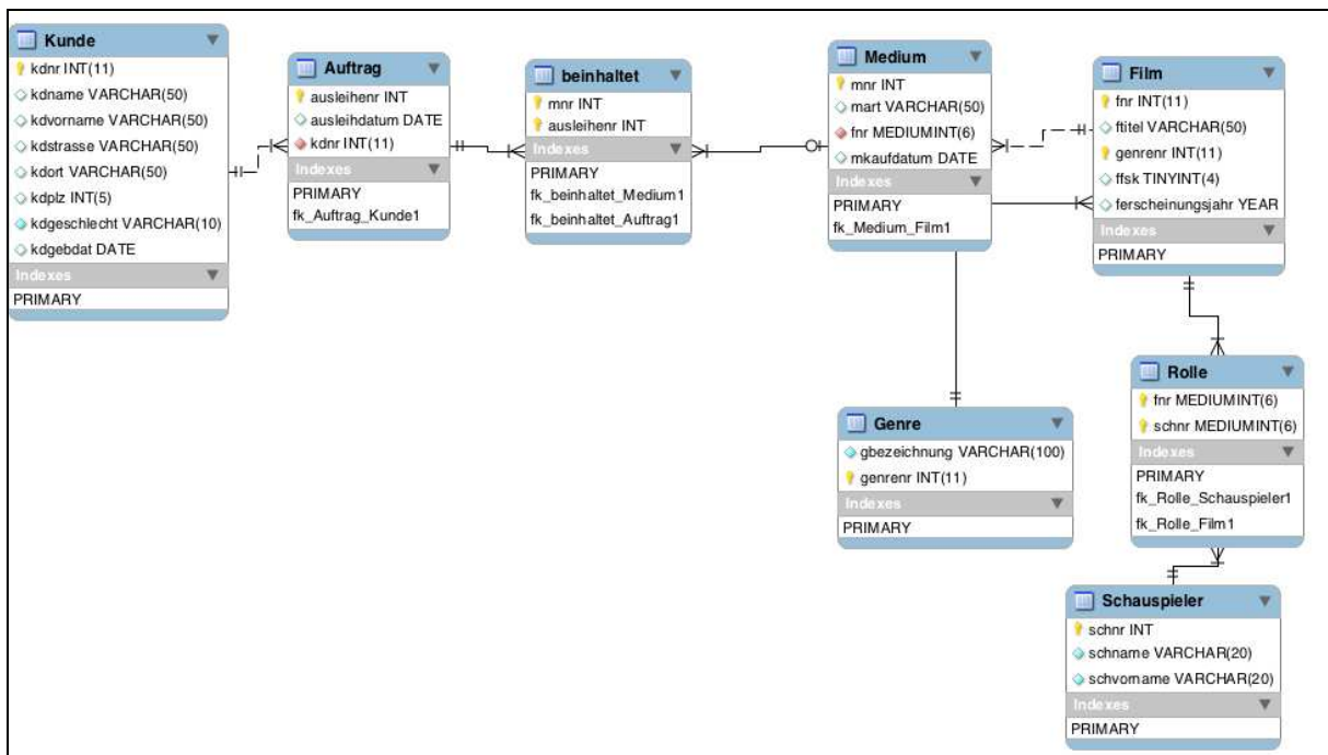
Modell der Datenbank mittels „MySQL workbench“ erzeugt
