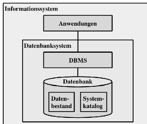
Modell eines Datenbanksystems
