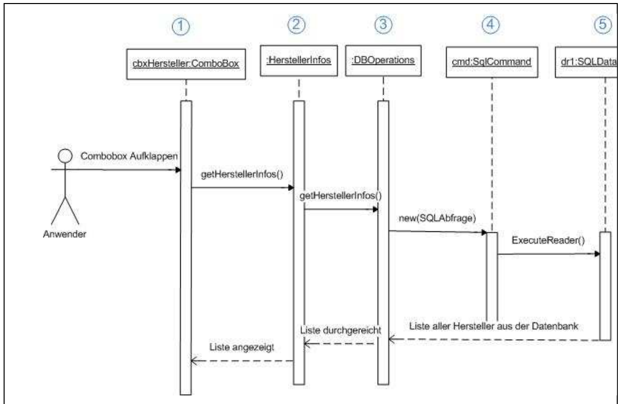
Sequenzdiagramm: HerstellerAnzeigen
